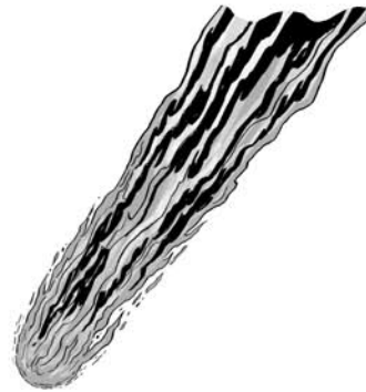
INSLAG METEORIET
